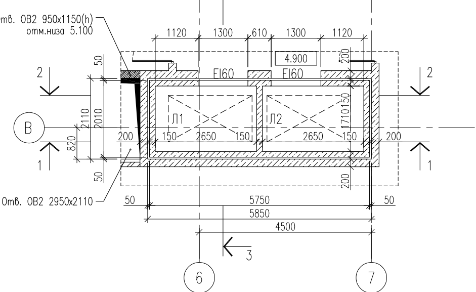
ФРАГМЕНТ ПЛАНА НА ОТМЕТКЕ 4.900
