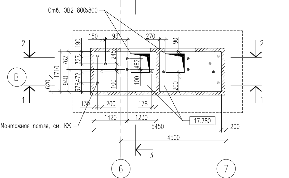
ПЛАН ПОКРЫТИЯ ШАХТЫ НА ОТМЕТКЕ 17.780
