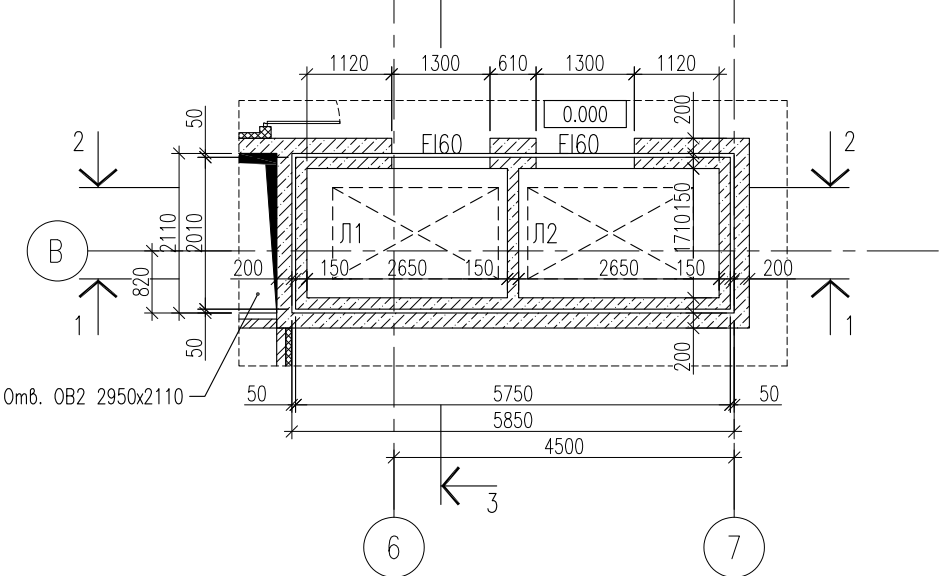
ФРАГМЕНТ ПЛАНА НА ОТМЕТКЕ 0.000
