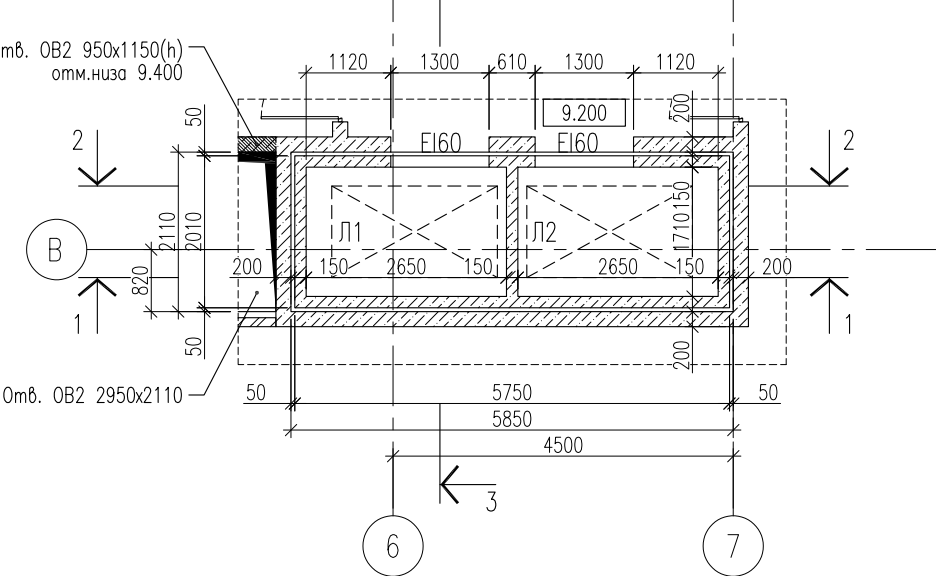
ФРАГМЕНТ ПЛАНА НА ОТМЕТКЕ 9.200
