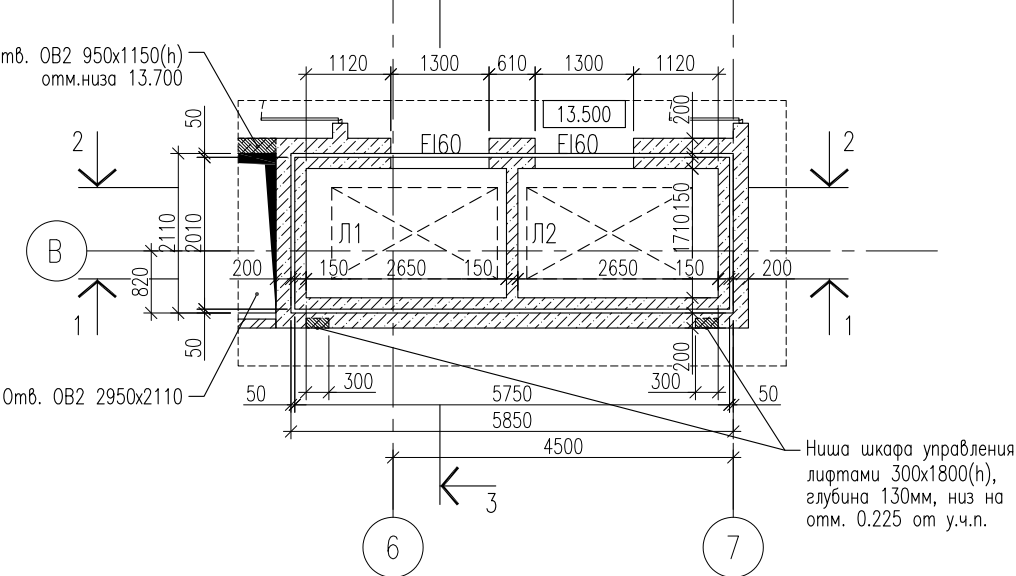
ФРАГМЕНТ ПЛАНА НА ОТМЕТКЕ 13.500
