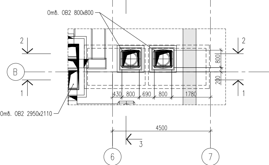
ФРАГМЕНТ ПЛАНА КРОВЛИ
