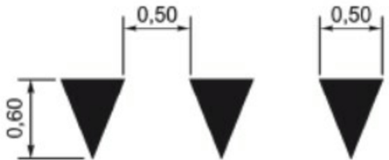
Горизонтальная разметка N1.13 по ГОСТ Р 51256–2018, цвет белый
