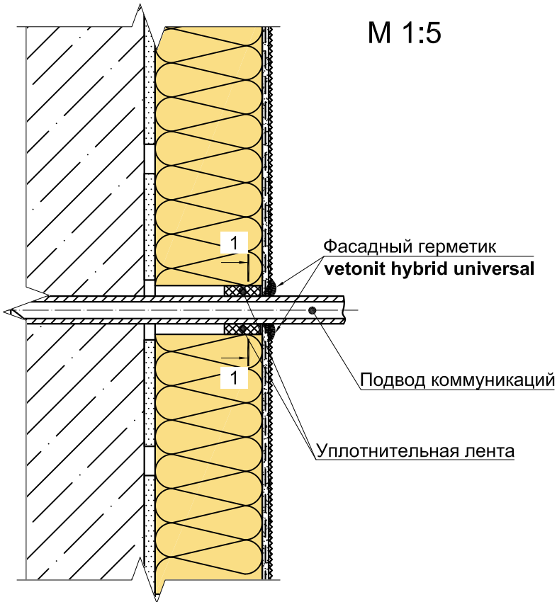
Разрез 1-1
