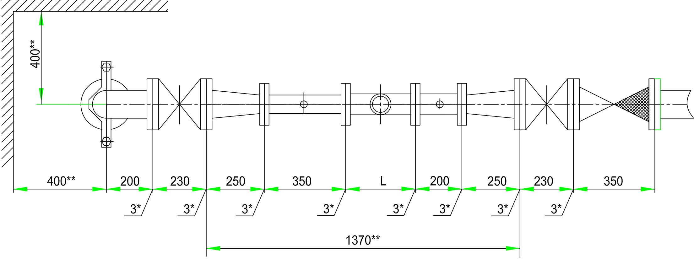
Установка счетчика \text{du}=65 \text{ мм} в водомерном узле линии на вводе диаметром 100 мм.
